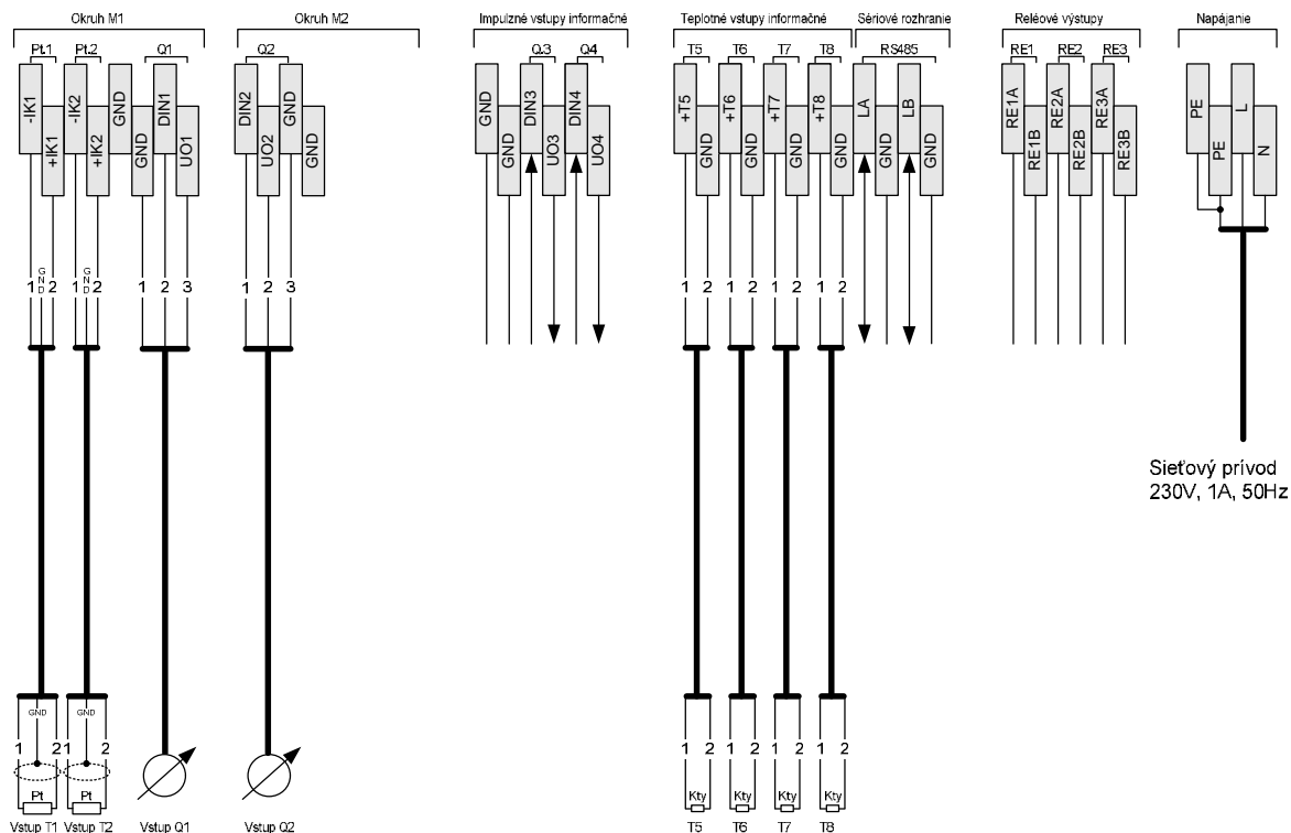
MAXTRONIC 15S - svorkové prepájanie
